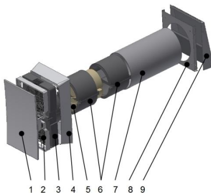
SEVi 160DUO MINI Bauteilzeichnung
