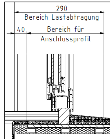
Bereich Fenstereinstand
