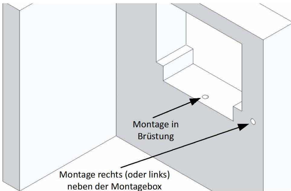
Positionierungsmöglichkeiten Netzteil
