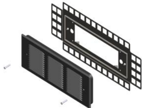
Montage Abdeckblech
