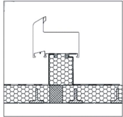
Fensterrahmen mit passendem Anschlussprofil
