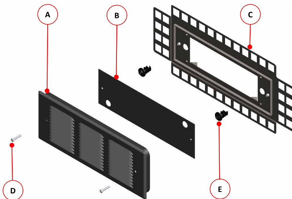
Komponenten Set Wetterschutzgitter
