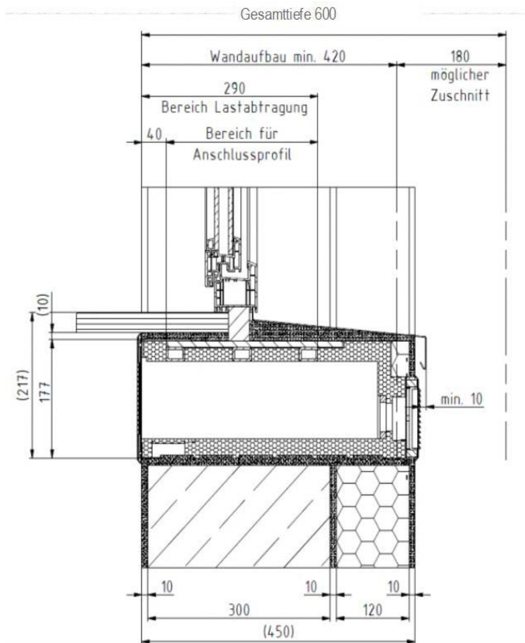
Schnitt Einbausituation Montagebox
