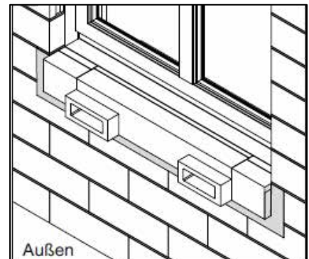
Außenabdichtung Montagebox
