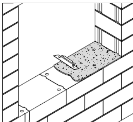
Höhenausgleich herstellen
