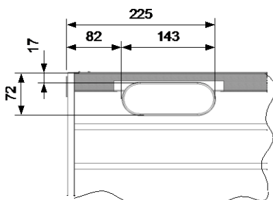
Lageskizze Unterseite Montagebox mit Nebenraumanschluss
