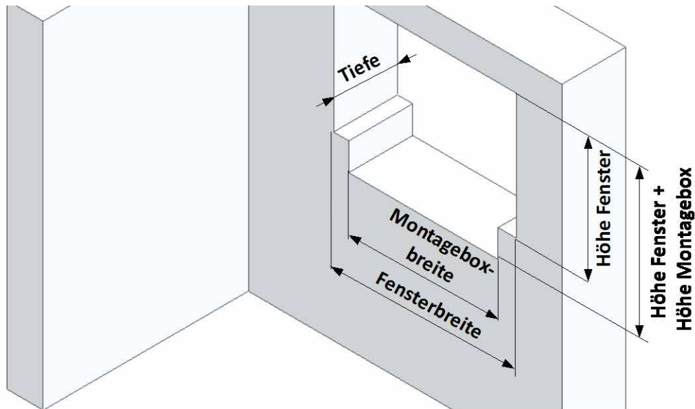
Einbauöffnung
