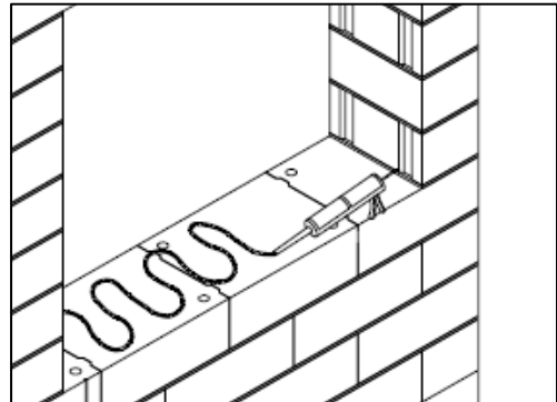
Herstellen Mörtelbett/Auftragen Montageschaum
