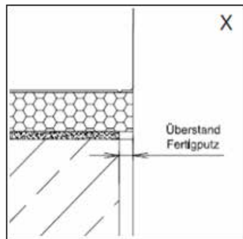
Montagebox bündig zum Innenputz ausrichten
