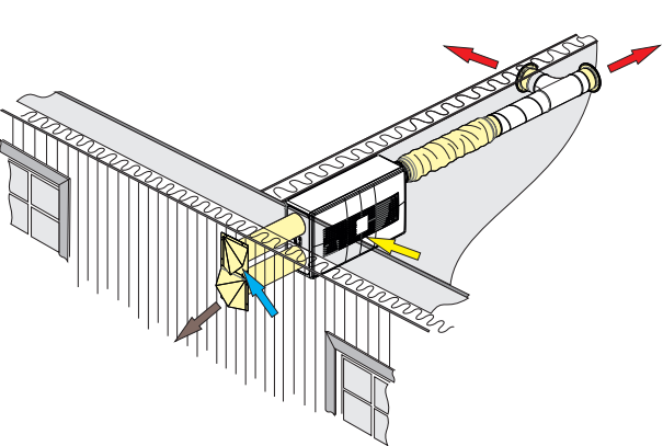
Pax Eos basmontage med tillbehören ytterväggssats, ljuddämpare och två tilluftsdon.
